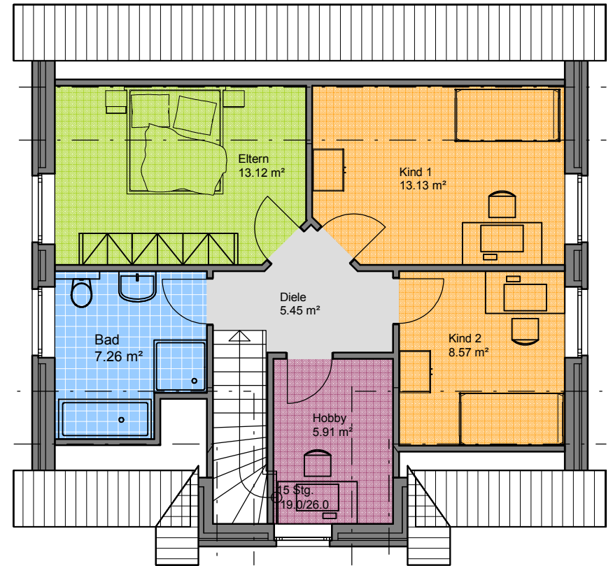
Dachgeschoss
