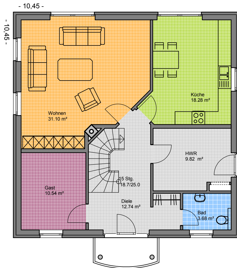
Erdgeschoss
