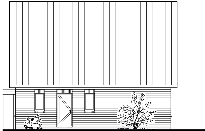
NORD OST ANSICHT
